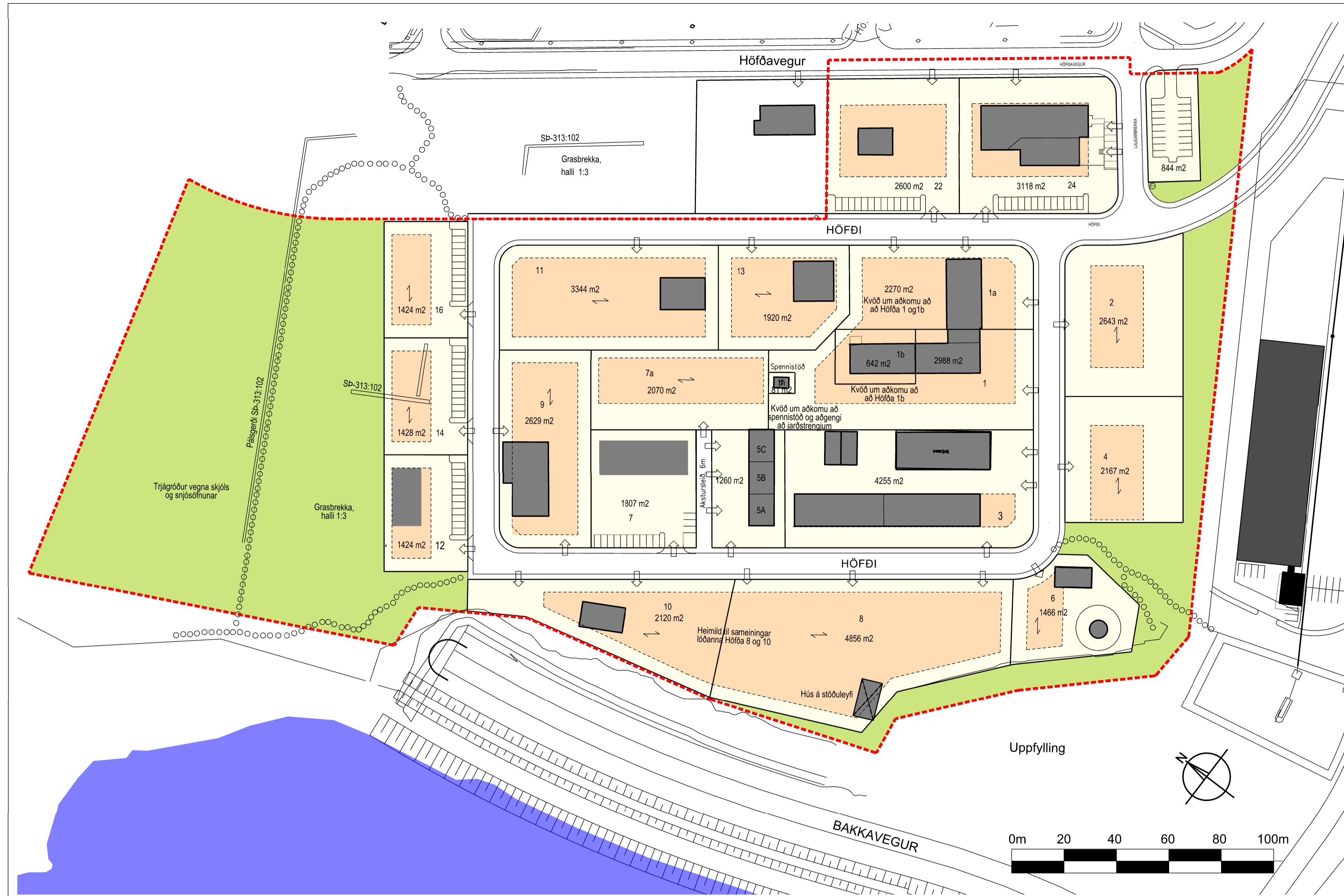
DEILISKIPULAG HÖFÐI, SVÆÐI A2 MKV. 1:1000
